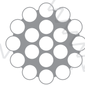
Hauban/Trapèze Shroud/Trapeze 1x19 monotoron
